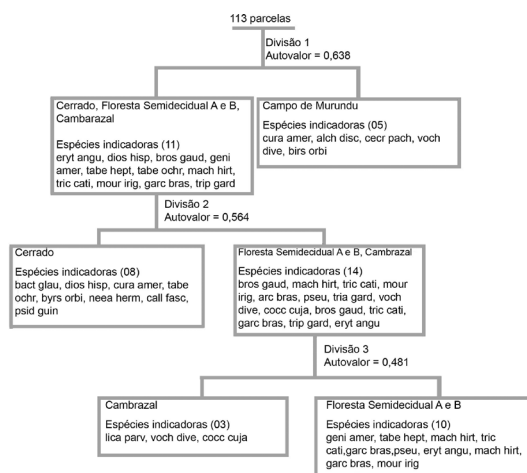
Figura 5 – An lise de TWISPAM para divis es das fitofisionomias em rela o  s esp cies indicadoras, com base nos dados de presenç a e aus ncia no Pantanal de Pocon , Mato Grosso.
