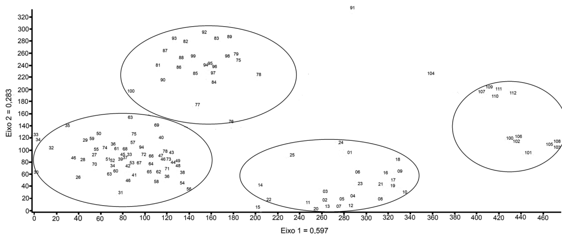
Figura 4 – Ordenação obtida para os dois primeiros eixos da análise de correspondência distendida (DCA), com base nos dados de abundância das espécies por subparcela, Pantanal de Poconé, Mato Grosso.
